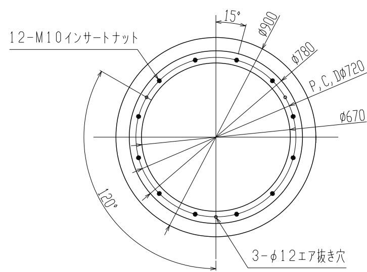
A-A断面図
