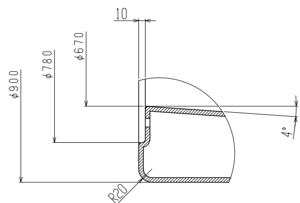
B部詳細図 (S=3:1)
