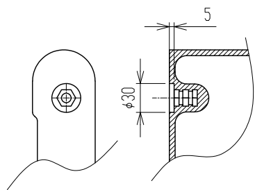
インサート部詳細 (S=1/15)
