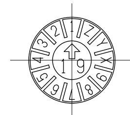
デートマーク詳細 (S=1/1)
