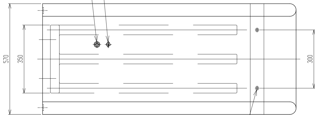
2-M10 SUS インサート (有効深サ15mm)
