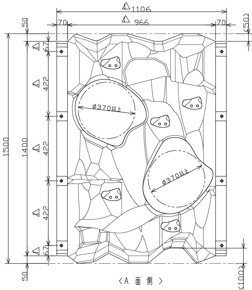
正面図 S=1/10
