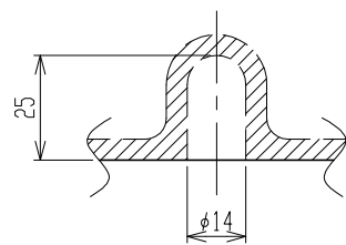
離形ピン詳細図
