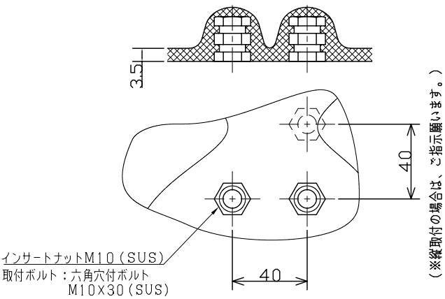
グリップ取付部詳細図
