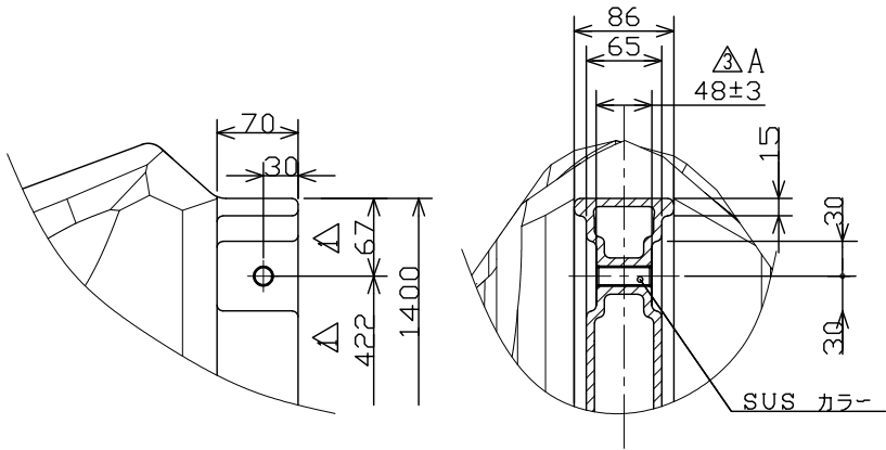
支柱取付部詳細図
