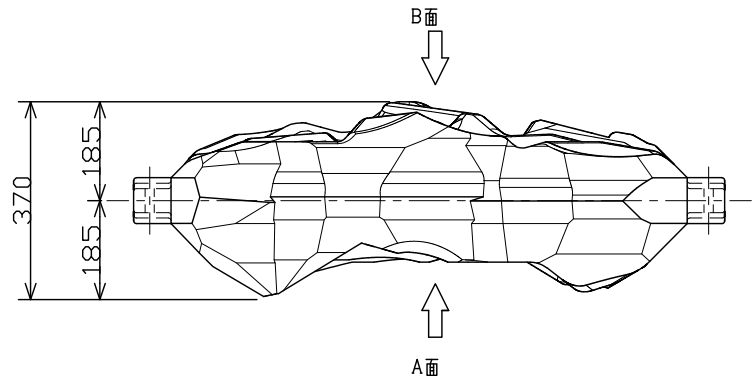
平面図 S=1/10
