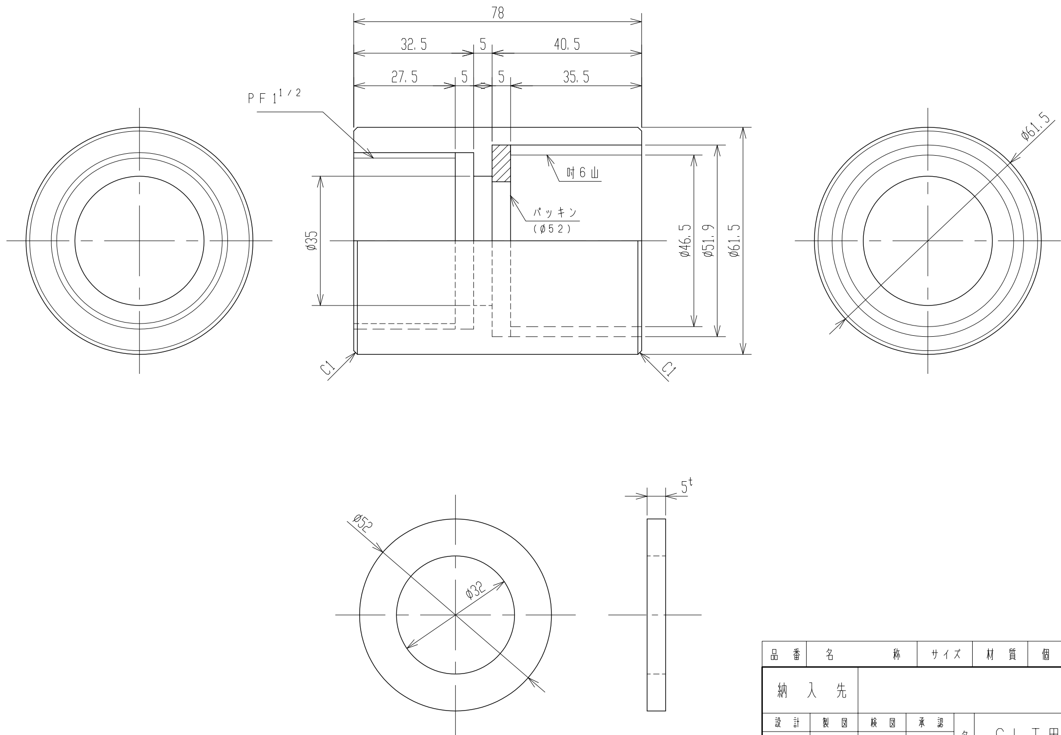
パッキン詳細 (NR)
