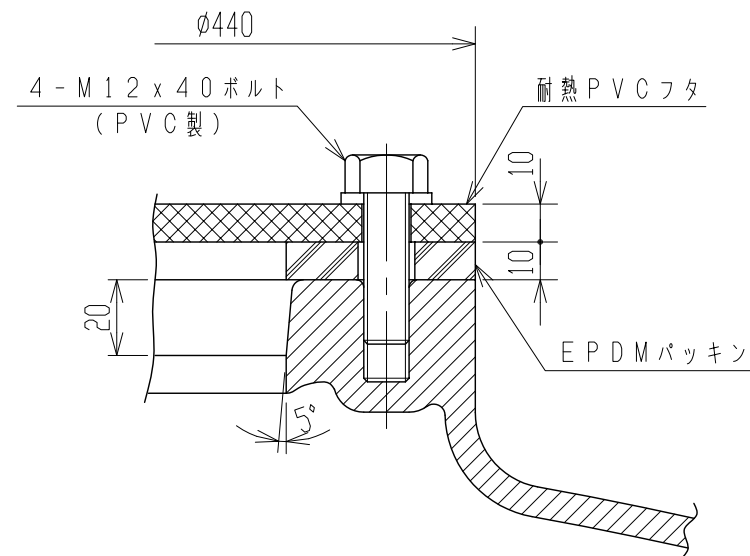
密閉マンホール詳細図 (S=1:2)
