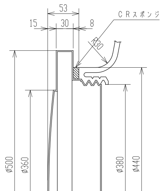
A 部 断 面 ( S = 1 / 4 )
