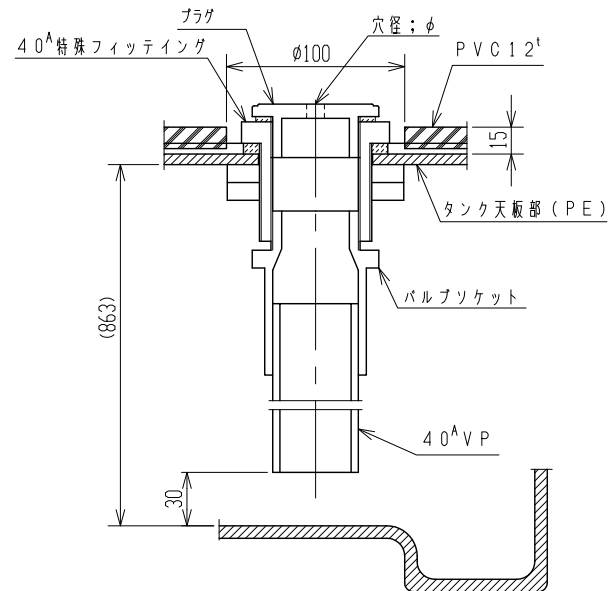
ポンプサクション口詳細 (S=1/3)
