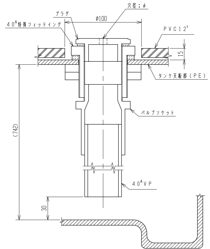
ポンプサクション口詳細 (S=1/2)
