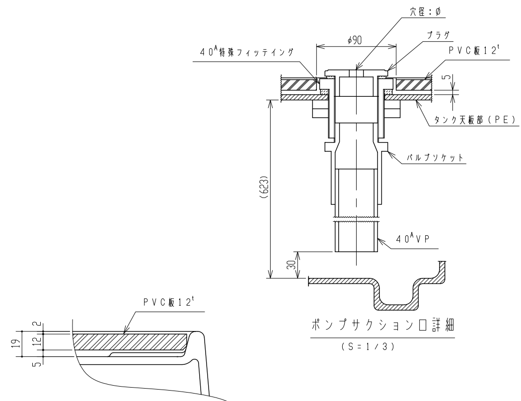
B部詳細図 S=1:2
