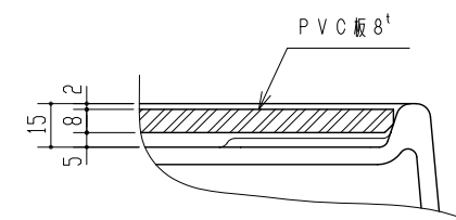
B 部詳細図 S = 1 : 2
