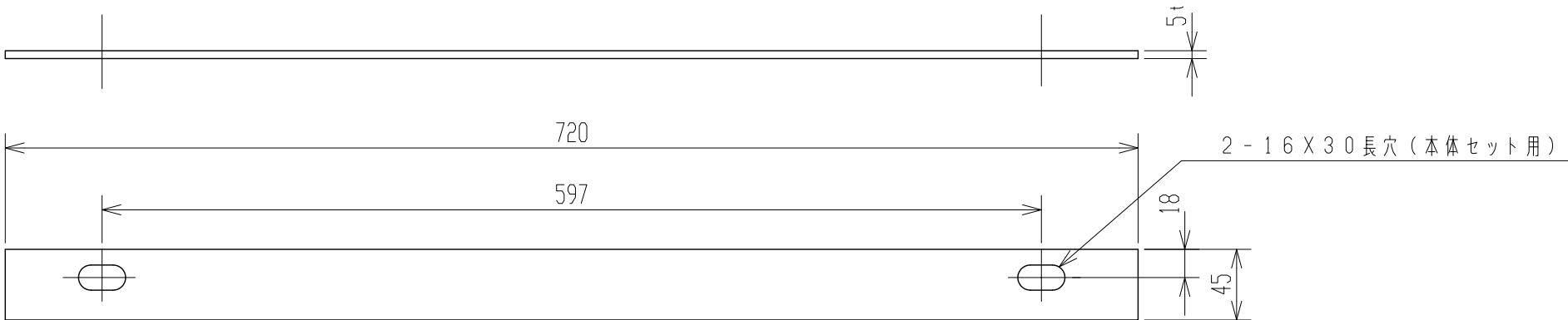
ブチルゴム t5
