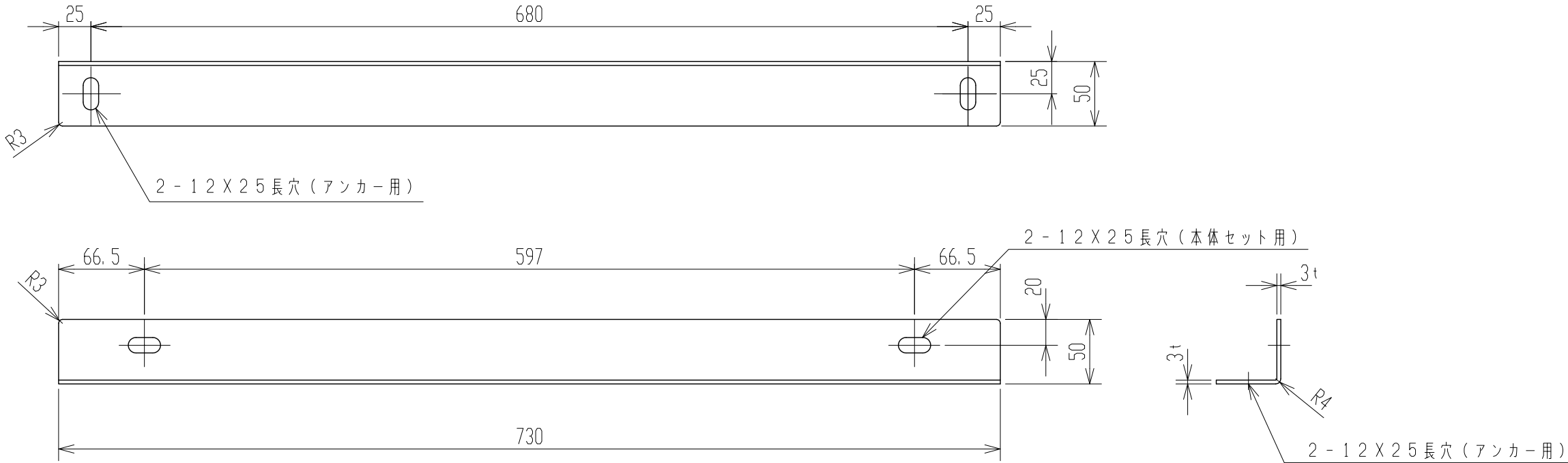
アンカープレート ( SUS 304 )
