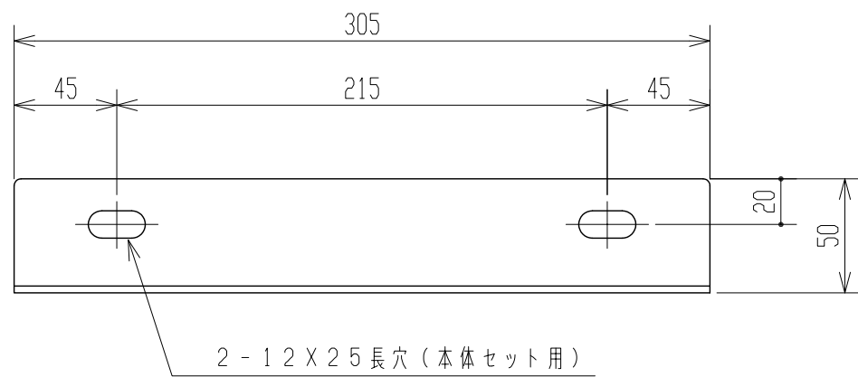
アンカープレート (SUS304)
