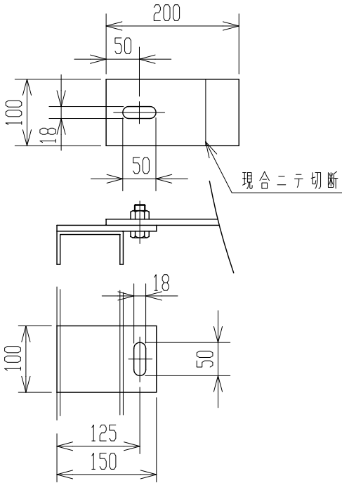
サポ-ト部詳細 (S=1/5)
