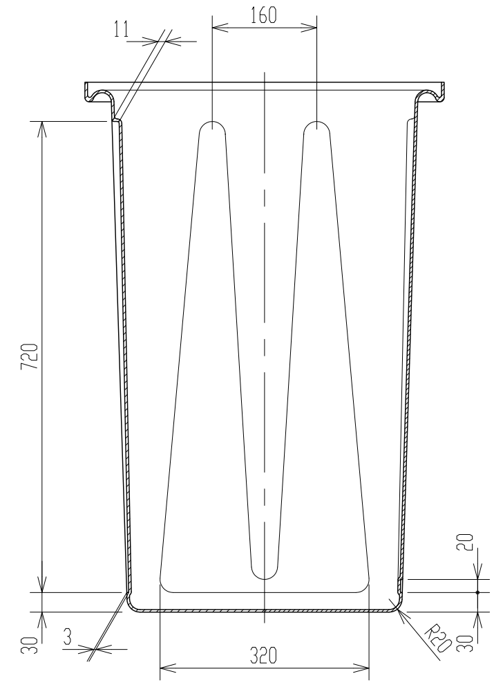
A - A 断面
