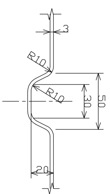
A-A断面 S=1:2
