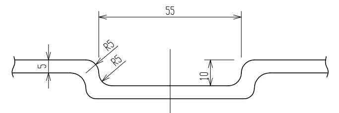
B - B 断面 (S = 1 / 1)
