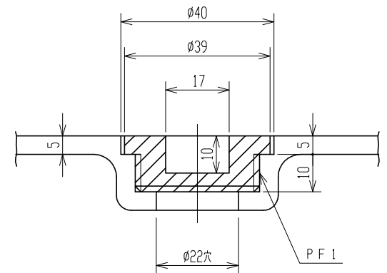
A 部断面詳細 (S = 1 / 1)
