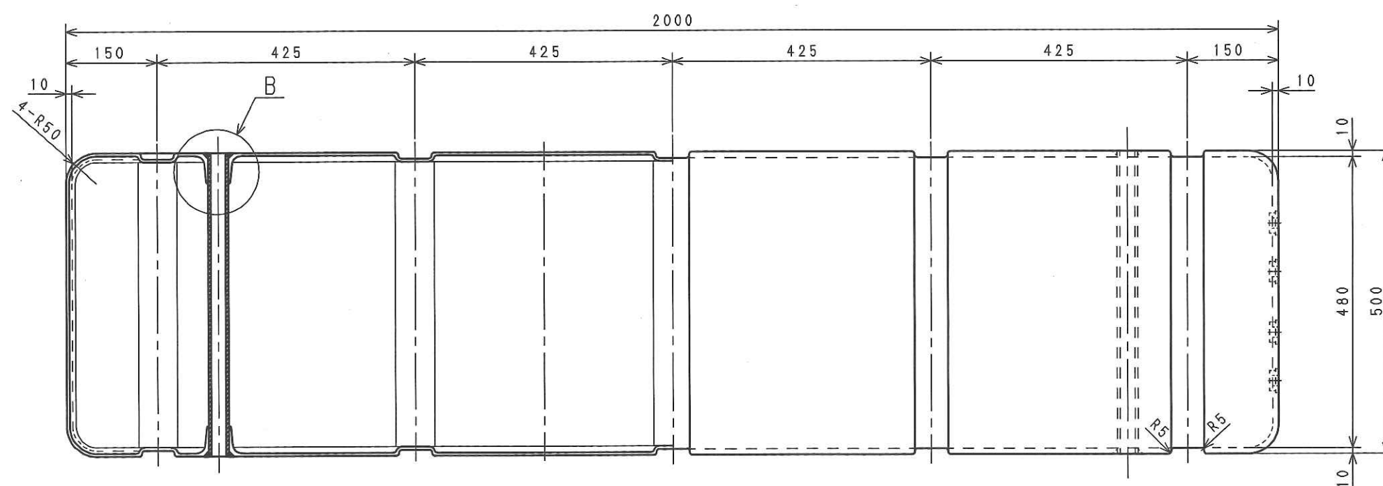
A-A断面
