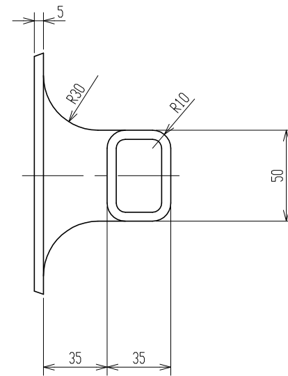
A-A断面 (S=1/2)
