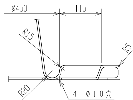
断面 A - A
