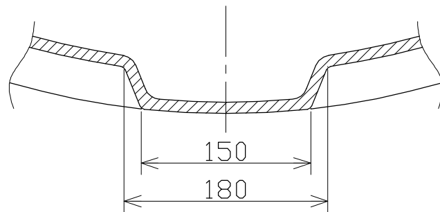
A-A断面
