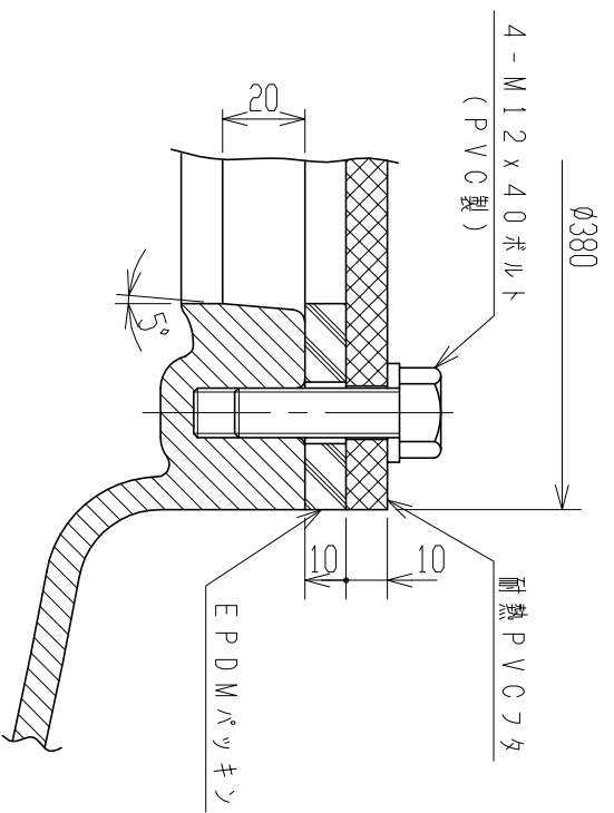
耐熱ツツホール詳細図 (S=1:2)
