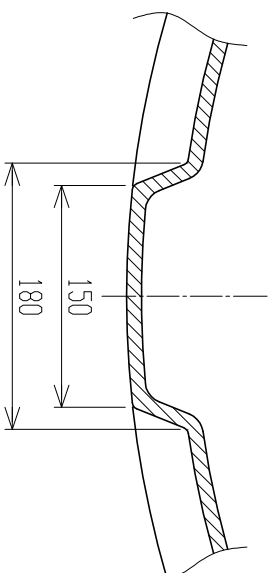
A-A断面 S=1:5
