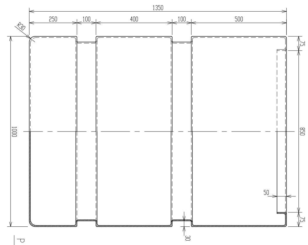
PE槽単体図
