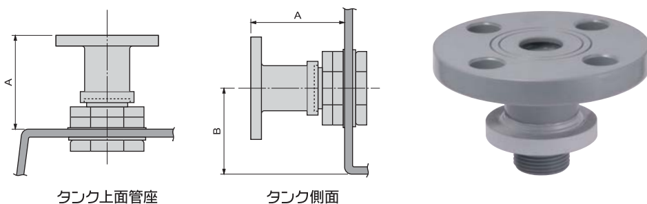
タンク上面管座
